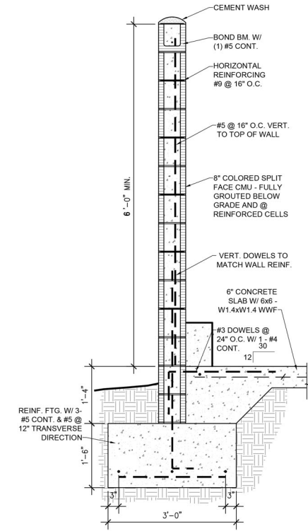
TRASH ENCLOSURE SECTION N.T.S.
