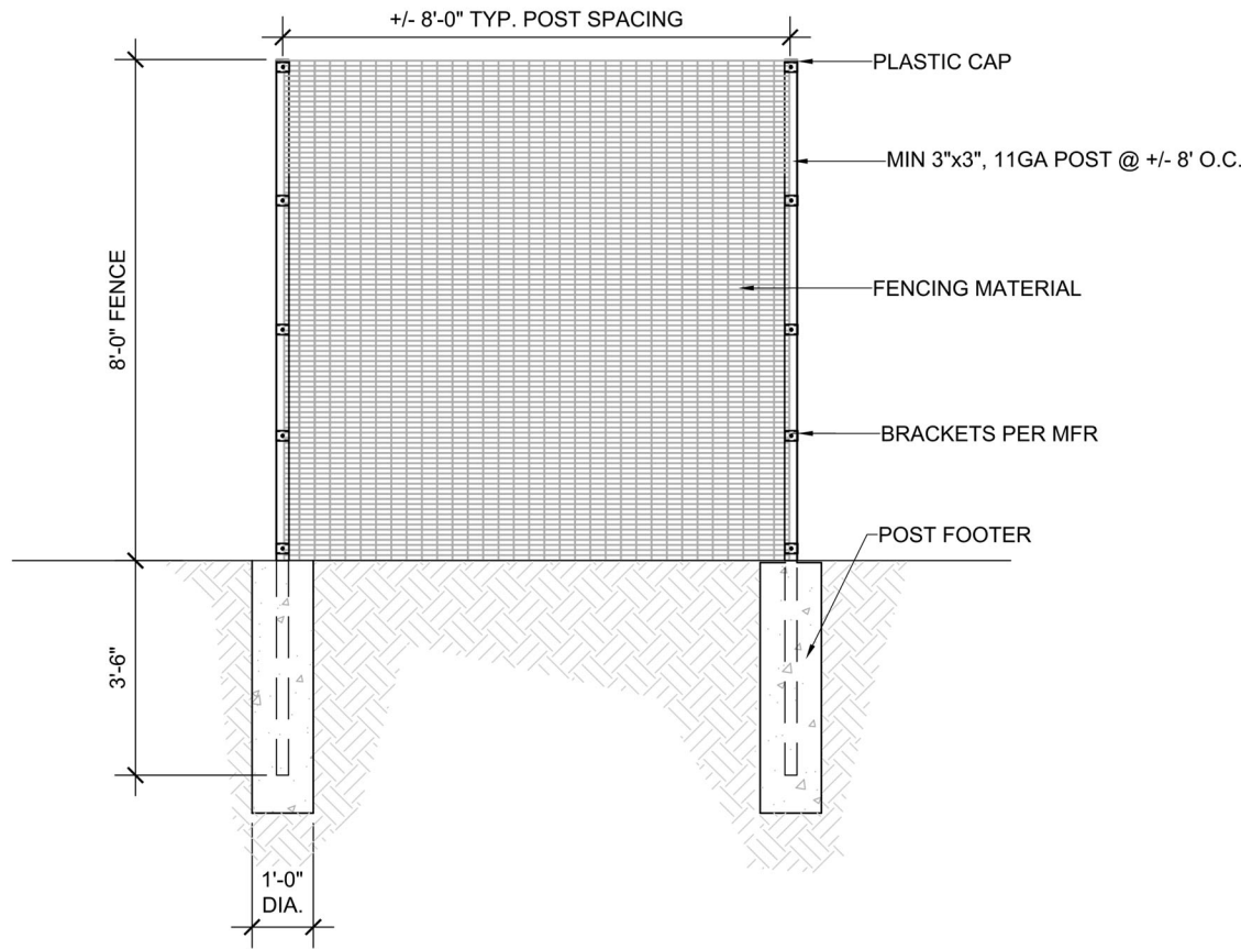
FENCE ELEVATION N.T.S.
