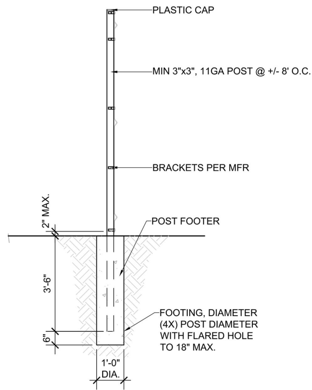
FENCE SECTION N.T.S.
